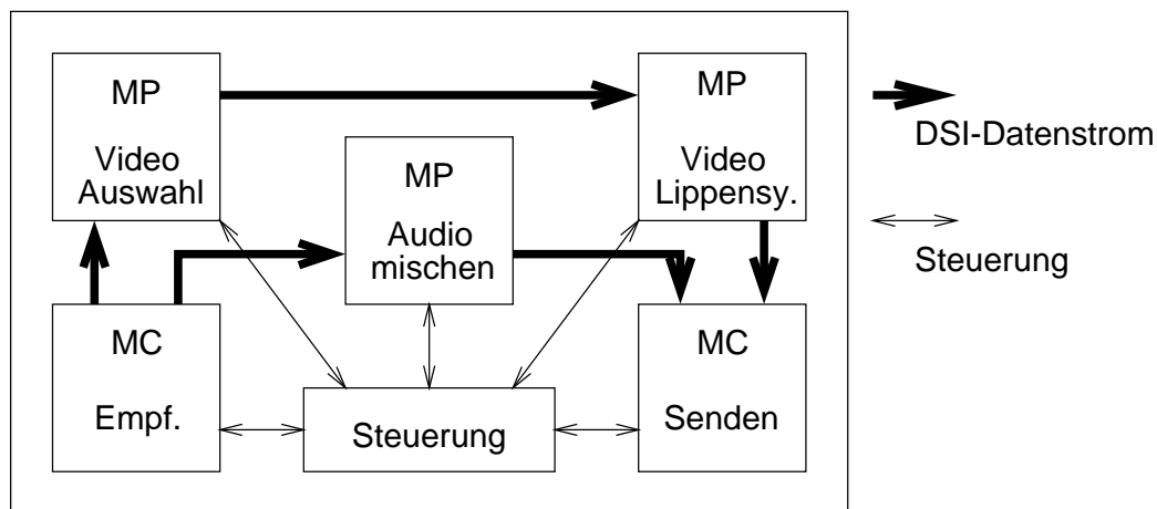
Abbildung 3.3.: Möglicher Aufbau eines MCU unter L4
