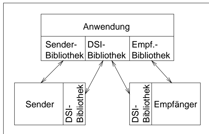
Abbildung 2.7.: Aufbau von DSI-Komponenten
