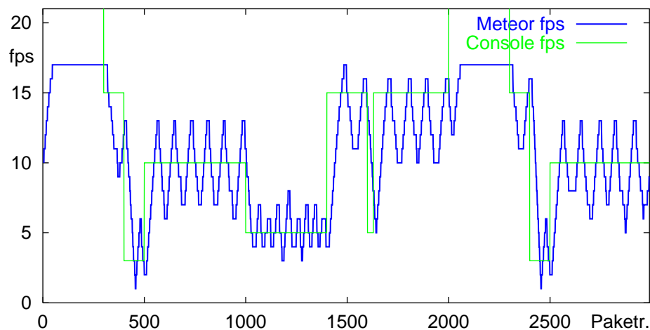
Abbildung 5.2.: Reaktion des Bildgenerators auf die Bildrate, die der Empfänger verarbeiten kann
