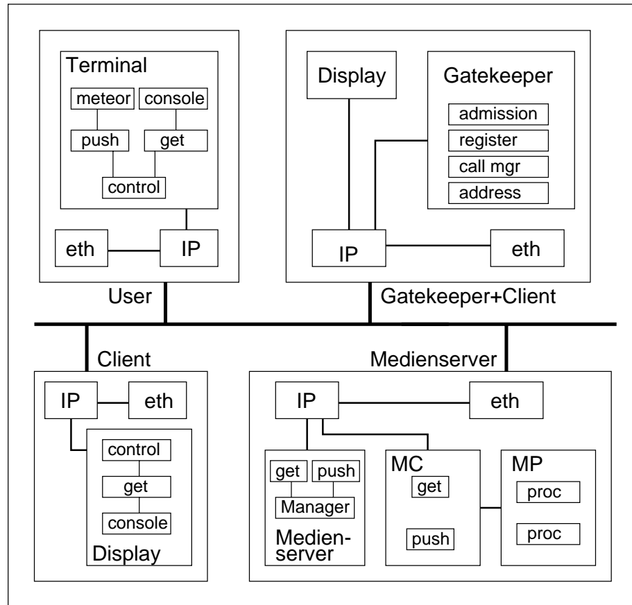
Abbildung 3.4.: Rechneraufteilung für eine mögliche Realisierung eines Videokonferenzsystems mit integriertem Medienserver
