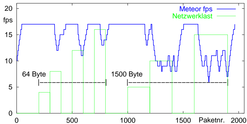
Abbildung 5.1.: Einfluß verschieden starker Netzlasten auf die Bildrate
