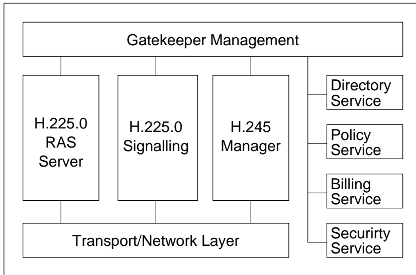
Abbildung 2.4.: Struktur eines Gatekeepers mit einigen Service-Einheiten für verschiedene Dienste
