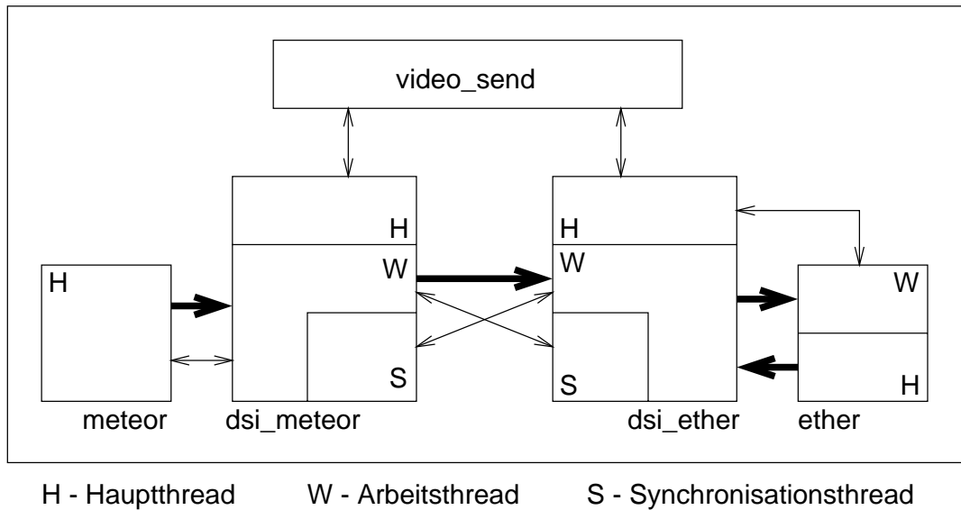
Abbildung 4.1.: Task- und Threadstruktur eines Rechners am Beispiel der Senderseite der DSI-Demonstration
