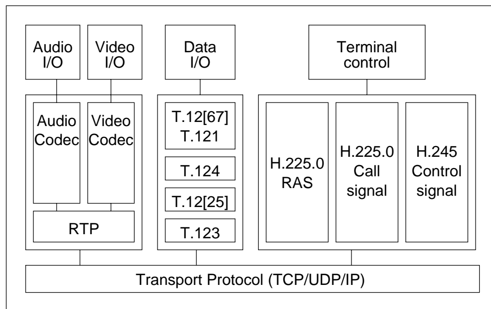
Abbildung 2.2.: H.323 Terminal Protokoll-Stack
