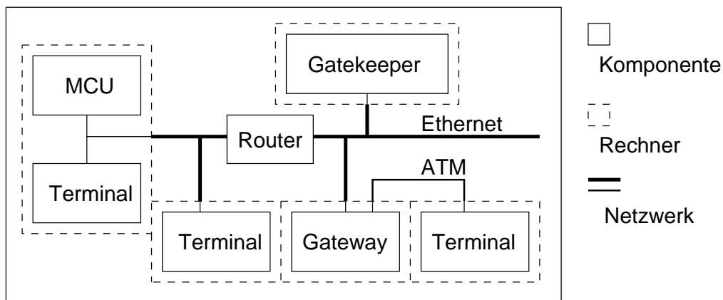
Abbildung 3.1.: H.323-Videokonferenz und deren mögliche Aufteilung auf 5 Rechner
