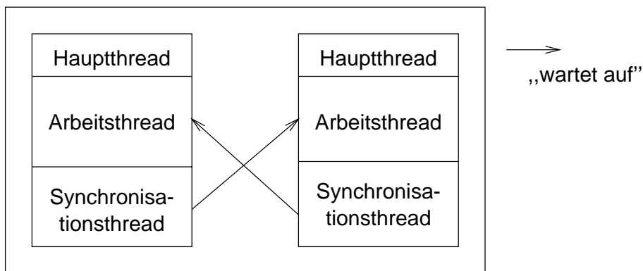
Abbildung 2.8.: Interaktion der Threads, die DSI vorschreibt
