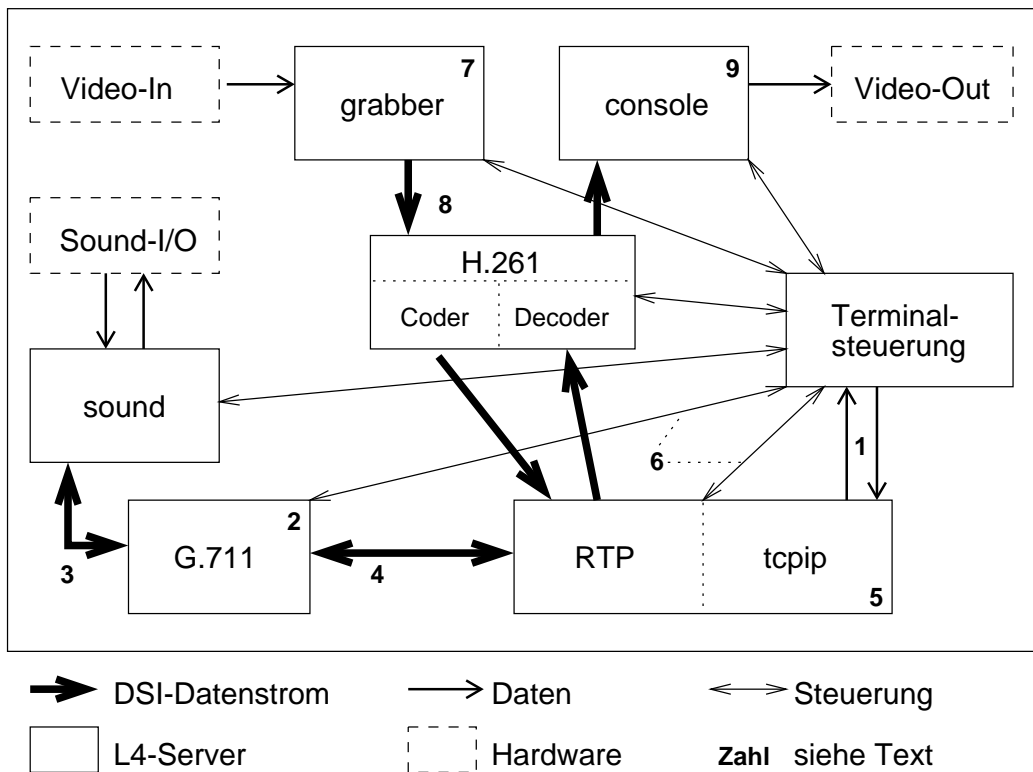
Abbildung 3.2.: Aufbau eines Nutzerterminals auf L4
