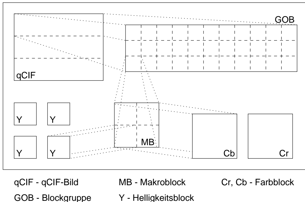
Abbildung 2.5.: Hierarchischer Aufbau eines Bildes im Format qCIF
