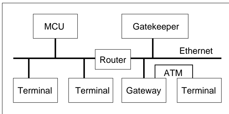
Abbildung 2.1.: Struktureller Aufbau eines möglichen H.323-Systems
